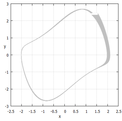
(f) SymReach.
