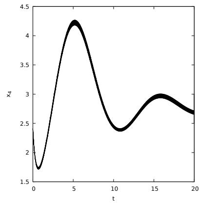
(e) Isabelle/HOL
