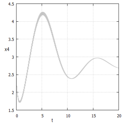
(f) SymReach
