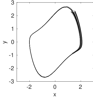
(a) CORA.
